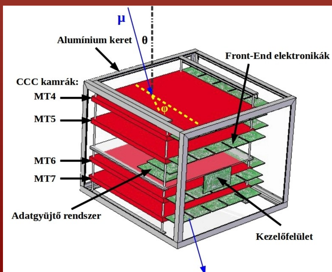
1. ábra: A müonteleszkóp szerkezete [1,2,3].
